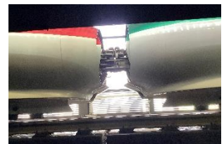
ホーム下から見える連結の様子
