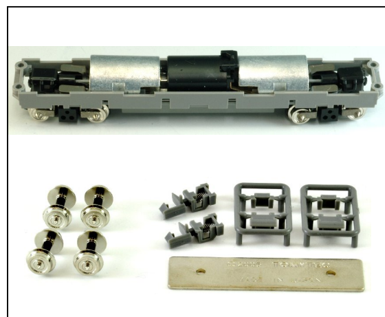
「デニ1300形専用動力ユニット」
