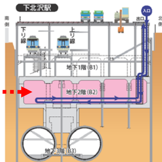
下北沢駅直下の横断面図(新宿側より)
