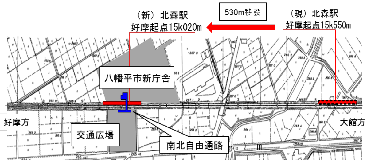
北森駅移設および南北自由通路設置概要図
