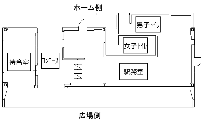
完成後の新駅舎平面図
