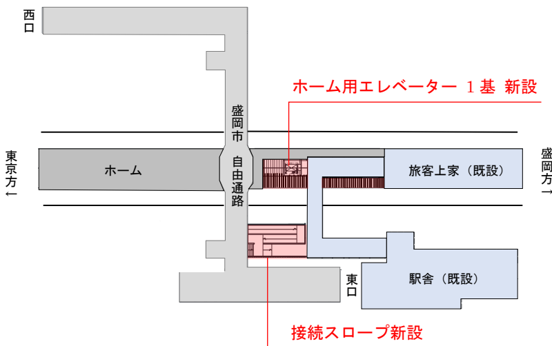
【平面計画】
