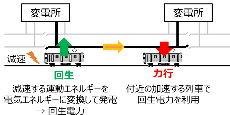
図1 回生電力の発電と利用
